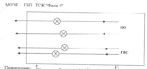
Схема учета тепловой энергии и теплоносителя (горячей воды) у потребителя Филевский бульвар, дом 34
