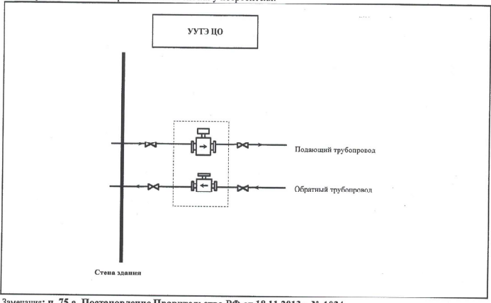
Схема учета тепловой энергии и теплоносителя у потребителя.
